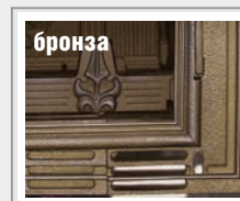
W10 - 14 кВт стекло - полукруглое вес - 156 кг, Ø 200 мм. ширина - 690 мм высота - 570 мм глубина - 440 мм
