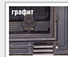
W11 - 14 кВт стекло - прямое вес - 141 кг, Ø 200 мм. ширина - 675 мм высота - 525 мм глубина - 410 мм
